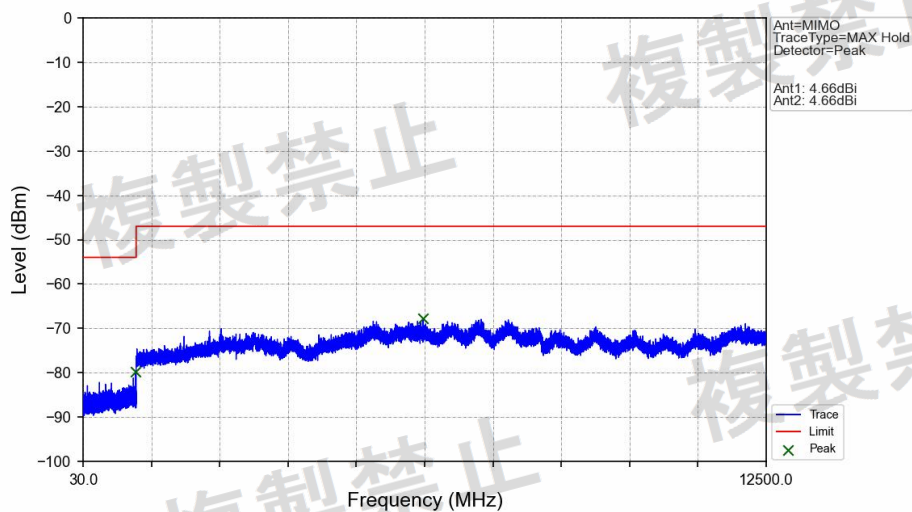
16QAM_2462.5MHz_MIMO_NTNV
