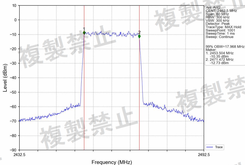
16QAM_2462.5MHz_Ant2_NTNV
