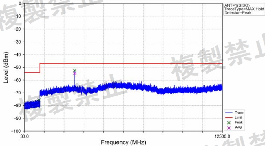
1M_2480MHz_Ant1_NTNV
