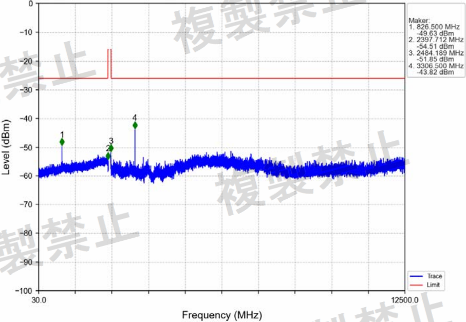
1M_2480MHz_Ant1_NTNV
