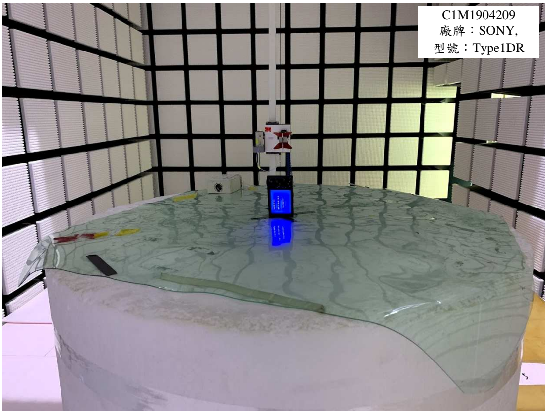
單機-側立
