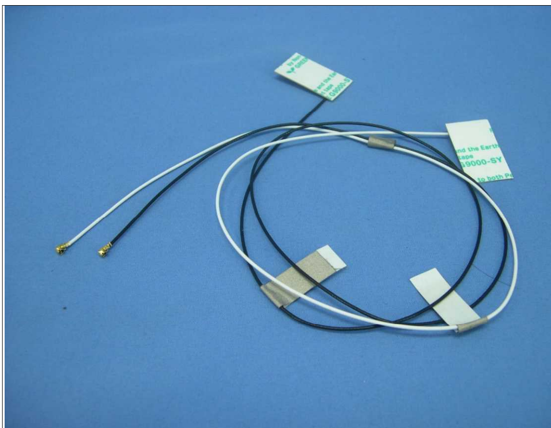
天線 26 TBN003 (Main) , TBN003 (Aux)
