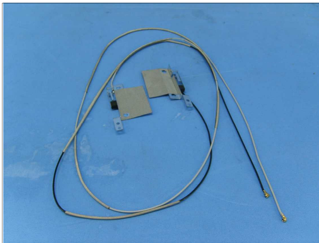
天線 5 ARW62WIPI01G (L) , ARW62WIP102G (R)
