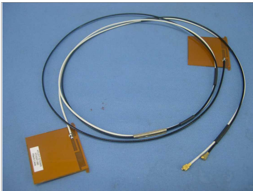
天線 21 HTL017 (Main) , HTL017 (Aux)
