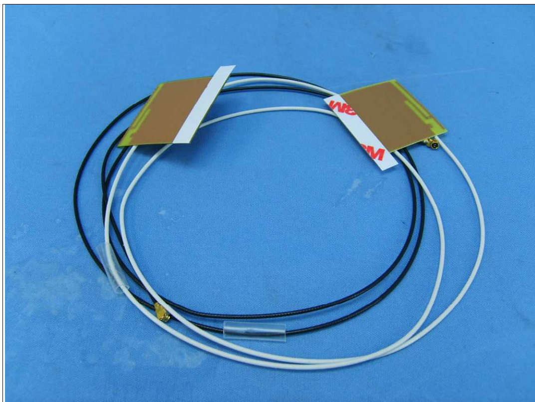
天線 13 81.EE215.016 (Main) , 81.EE215.016 (Aux)
