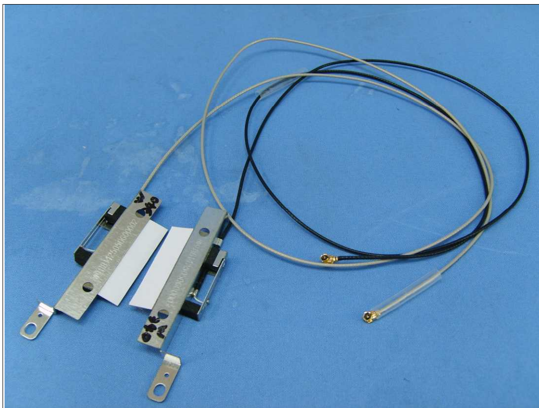
天線 15 B1425050G00003 (Main) , B1425050G00002 (Aux)
