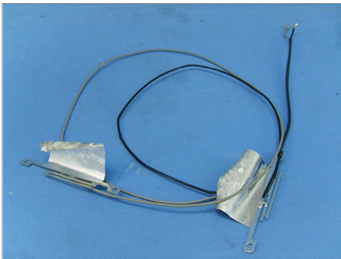
天線 7 WDAN-GQMA6001-DF (Main) , WDAN-GQMA6001-DF (Aux)
