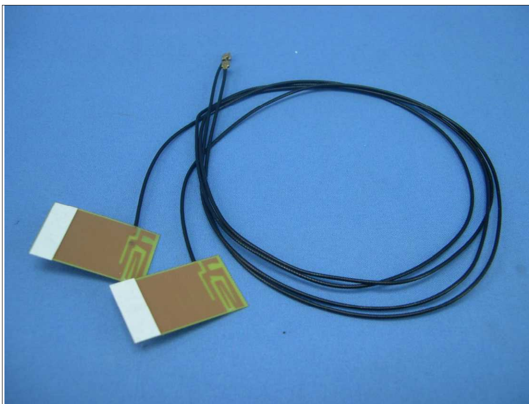
天線 22 WNC001 (Main) , WNC001 (Aux)
