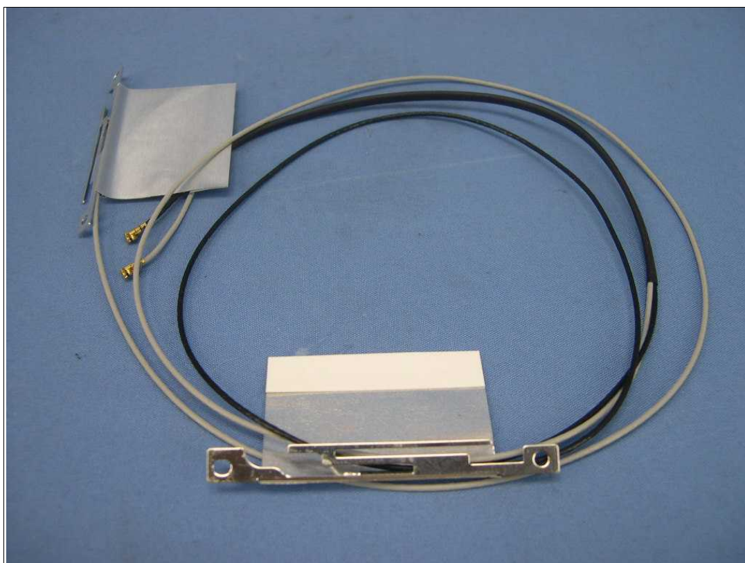
天線 2 DQ661500115(Main) , DQ661500115 (Aux)
