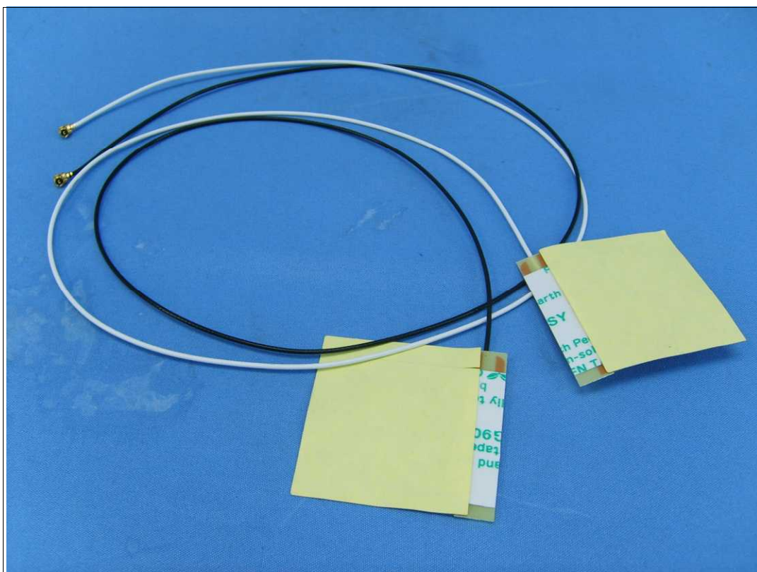
天線 16 ASAT 001 (Main) , ASAT 001 (Aux)
