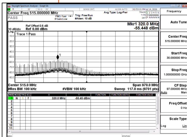
RX Below 1GHz BLE 1M 2402MHz
