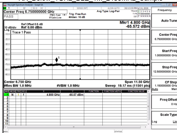
RX Above 1GHz BLE 1M 2480MHz
