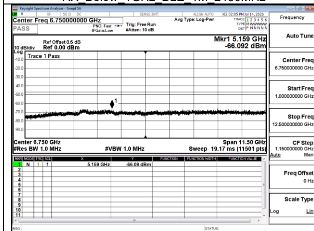
RX Above 1GHz BLE 1M 2402MHz
