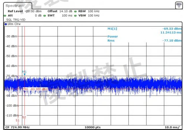
NTNV-11AC20-Ant2-5300-30~1000-PASS
