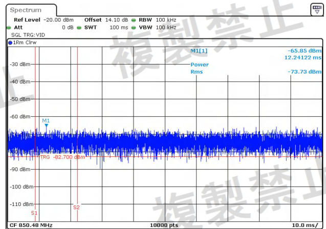
NTNV-11N40MIMO-Ant1-5270-30~1000-PASS
