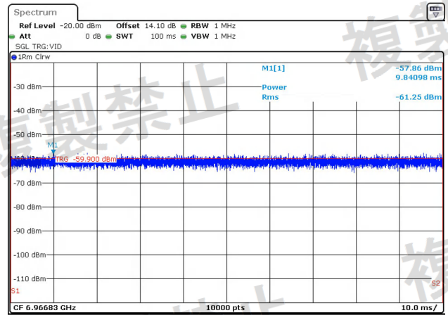
NTNV-11AC20-Ant2-5300-1000~26000-PASS
