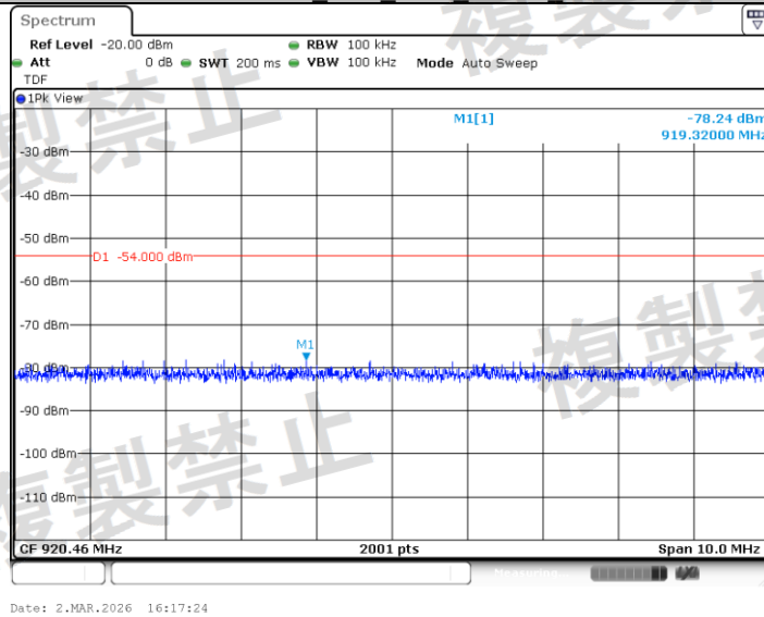
11N40MIMO_Ant1_2422_920.46_Ant1
