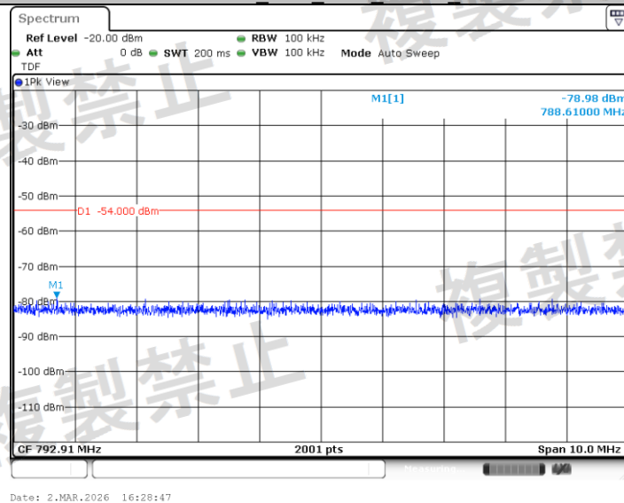
11N40MIMO_Ant0_2462_792.91_Ant0
