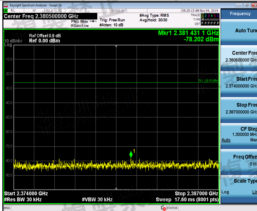
TNVL_2DH5_Ant1_2480_2374~2387
