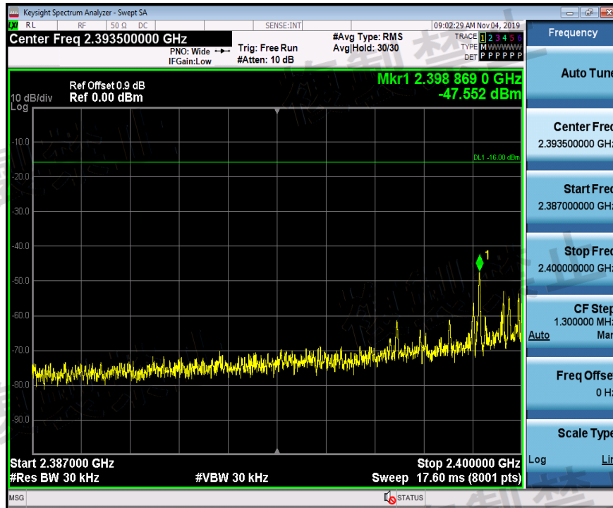
TNVL_3DH5_Ant1_2402_2387~2400
