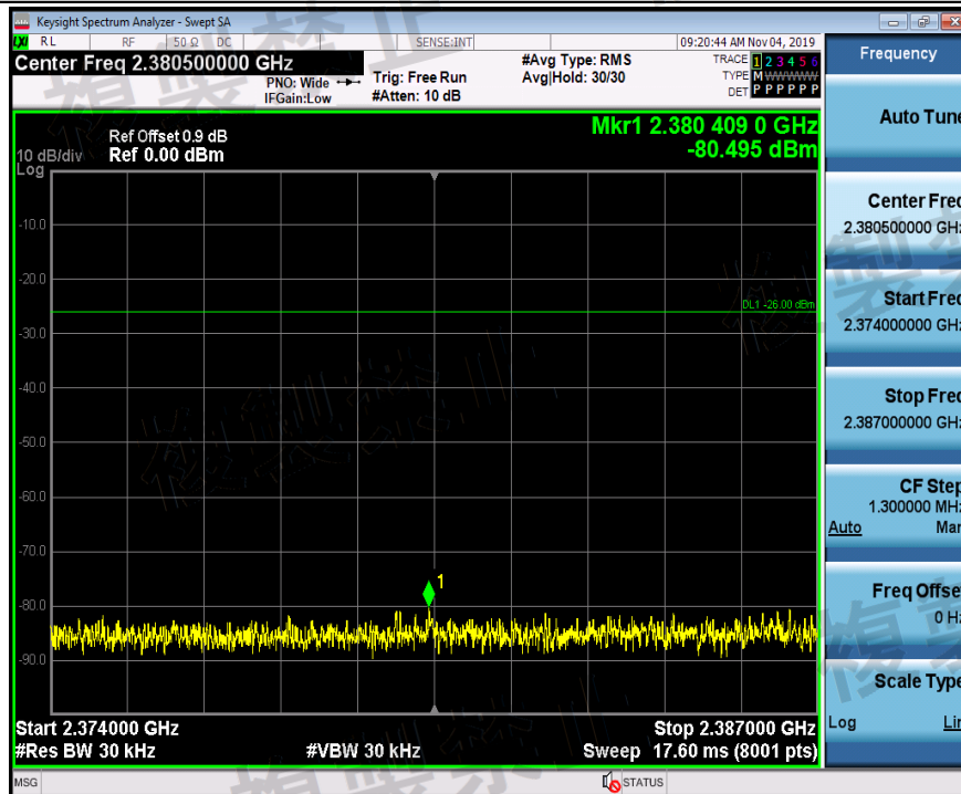
TNVL_DH5_Ant1_2480_2374~2387
