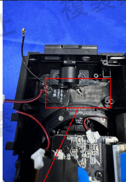
antenna
