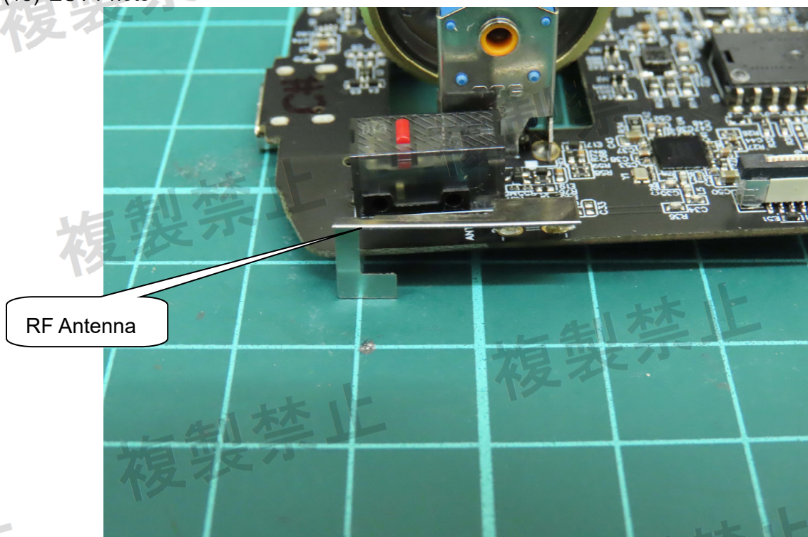
(13) EUT Photo
